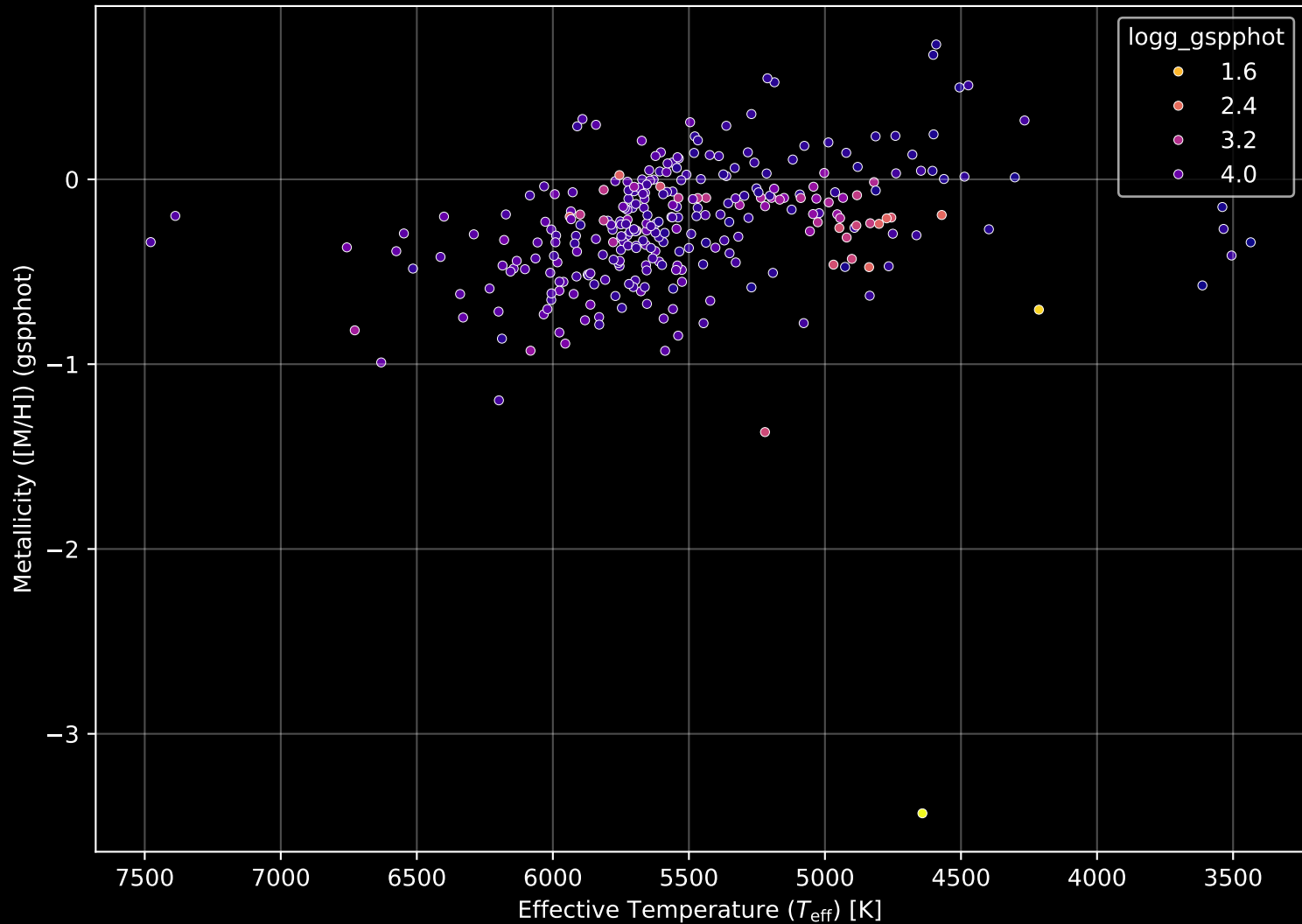
GALAH DR4 Field: [6927] Stellar Population Parameters (n= 298)
